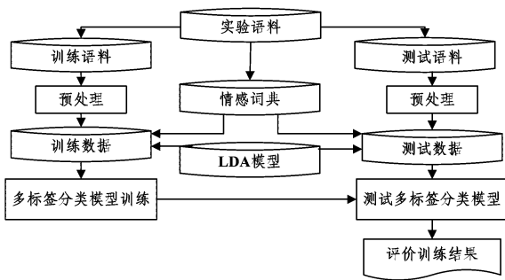
图 2 句的情感极性判断框架
