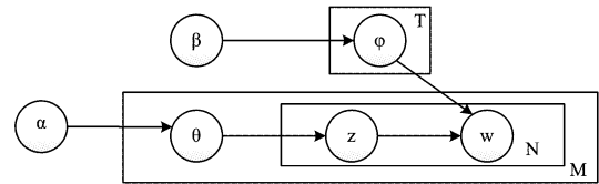
图 1 LDA 的图模型表示
