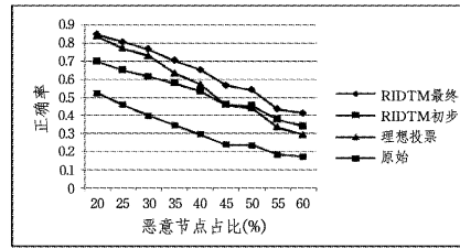
图5 算法正确率对比
