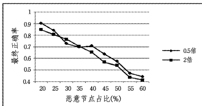
图4 算法针对不同攻击方式的正确率
