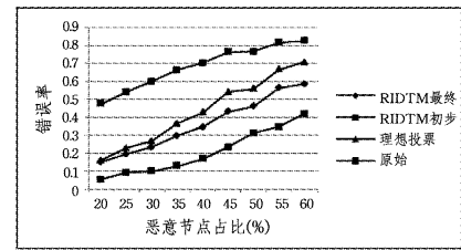
图6 算法错误率对比
