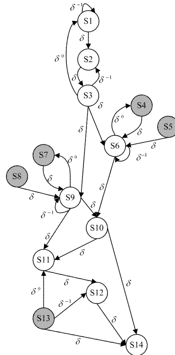
图 2 图 1 核心程序段对应的数据依赖图
