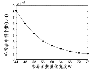
图3 参数 W 与哈希桶个数的关系
