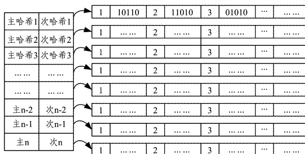
图2 单词(哈希值)映射链结构图
