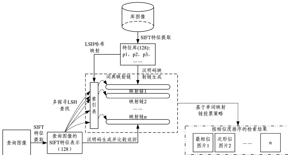
图1 基于哈希聚类 and 单词映射链投票的图像检索流程图
