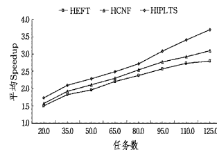
图 7 不同任务数下的加速比对比
