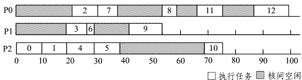
图 5 HEFT 算法调度甘特图
