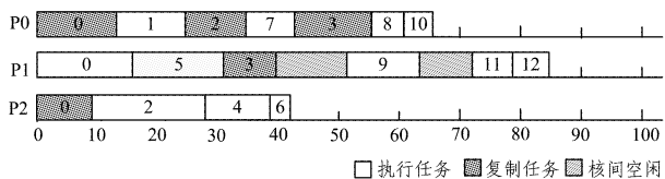
图 6 HCNF 算法调度甘特图
