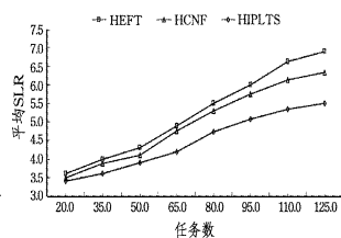
图 8 不同任务数下的 SLR 对比图
