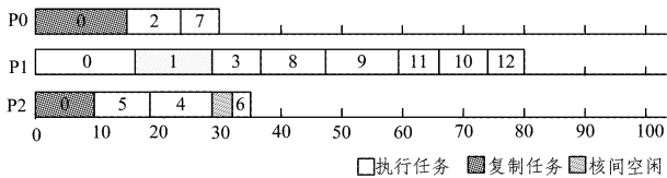
图 4 HIPLTS 算法调度甘特图
