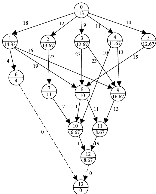
图 3 DAG 任务图
